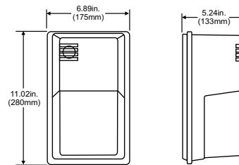
MIMWPK-277PC - 277V Photocell
